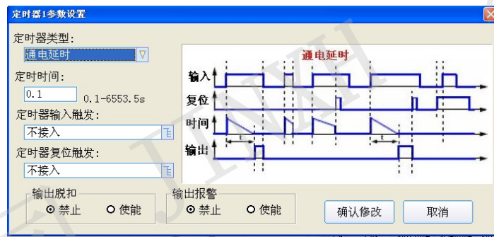
图 30 定时器
