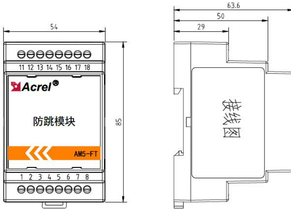
图 3 AM5-FT 尺寸图
