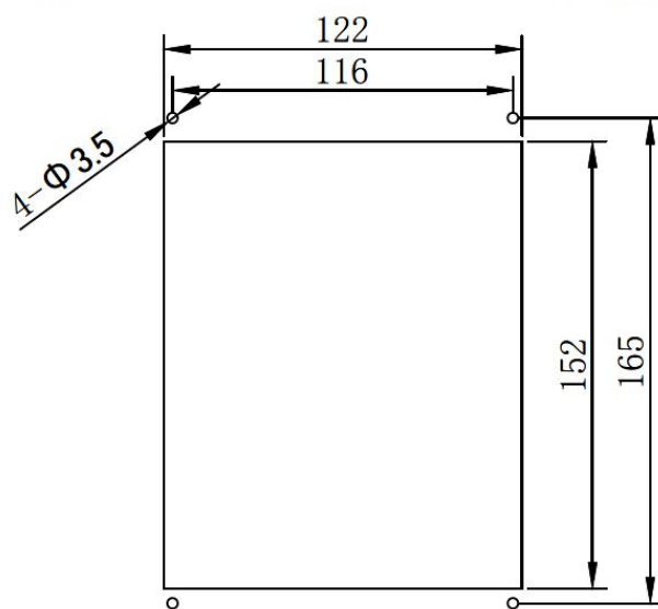
开孔尺寸
