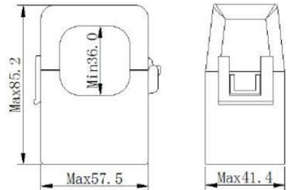
Φ 36mm
